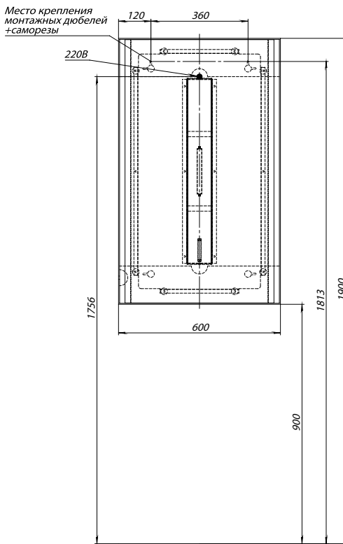
INFINITY 600X1000 ПРЯМОУГЛЬНОЕ. ВЕРТИКАЛЬНОЕ РАСПОЛОЖЕНИЕ
