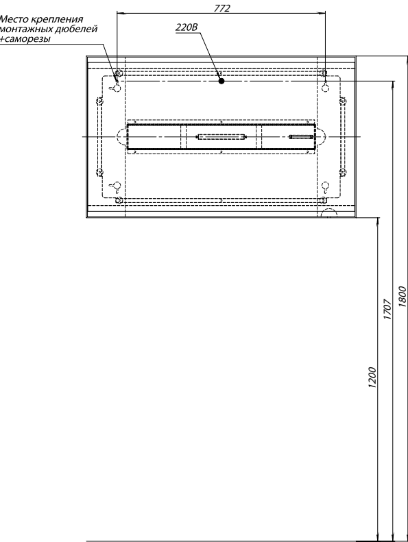
INFINITY 600X1000 ПРЯМОУГЛЬНОЕ. ГОРИЗОНТАЛЬНОЕ РАСПОЛОЖЕНИЕ
