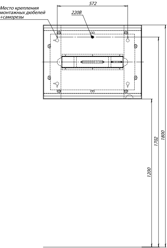
INFINITY 600X800 ПРЯМОУГЛЬНОЕ. ГОРИЗОНТАЛЬНОЕ РАСПОЛОЖЕНИЕ
