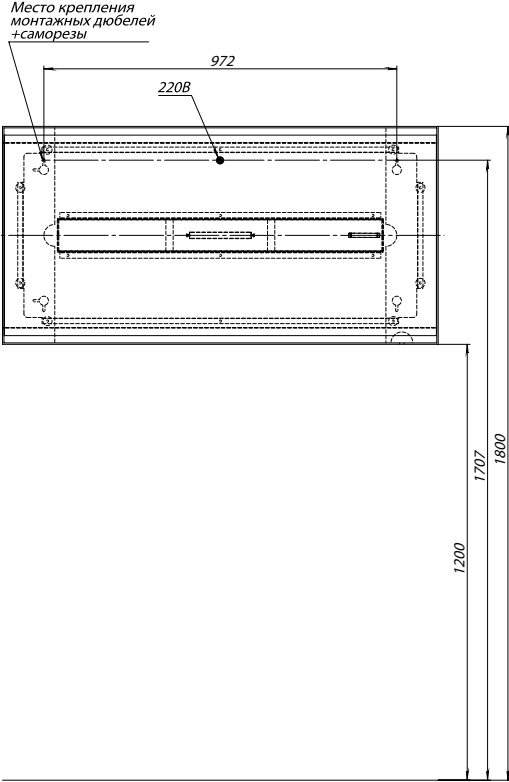
INFINITY 600X1200 ПРЯМОУГЛЬНОЕ. ГОРИЗОНТАЛЬНОЕ РАСПОЛОЖЕНИЕ
