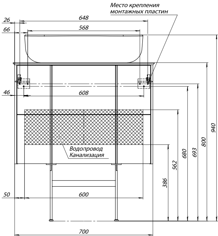
ТУМБА REALITY 71 СО СТОЛЕШНИЦЕЙ
